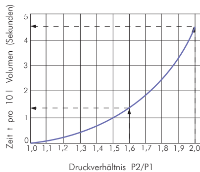
DUE 1600 A
